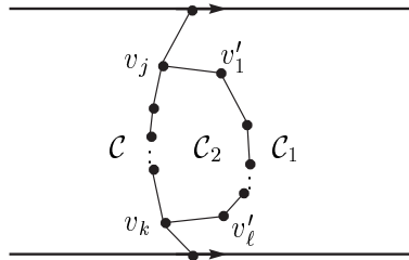
Fig. 4. Illustration of Lemma 12.
